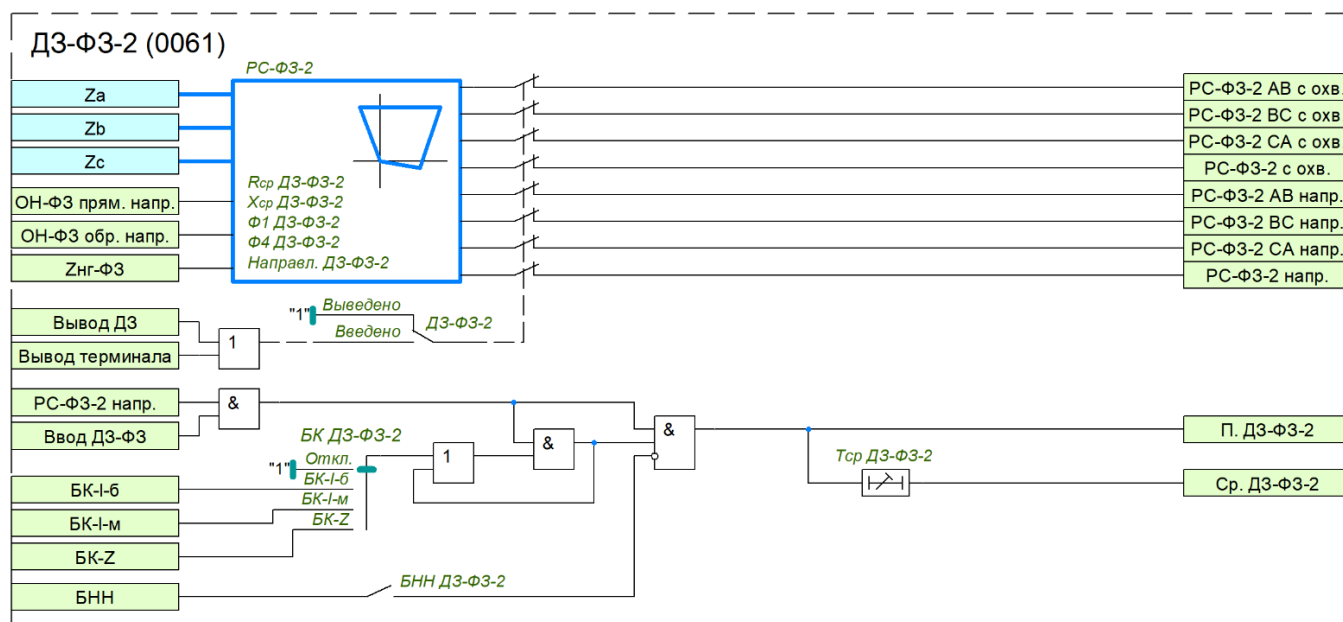
Рисунок 1.11 – Функциональная схема логики ДЗ-Φ3-2
